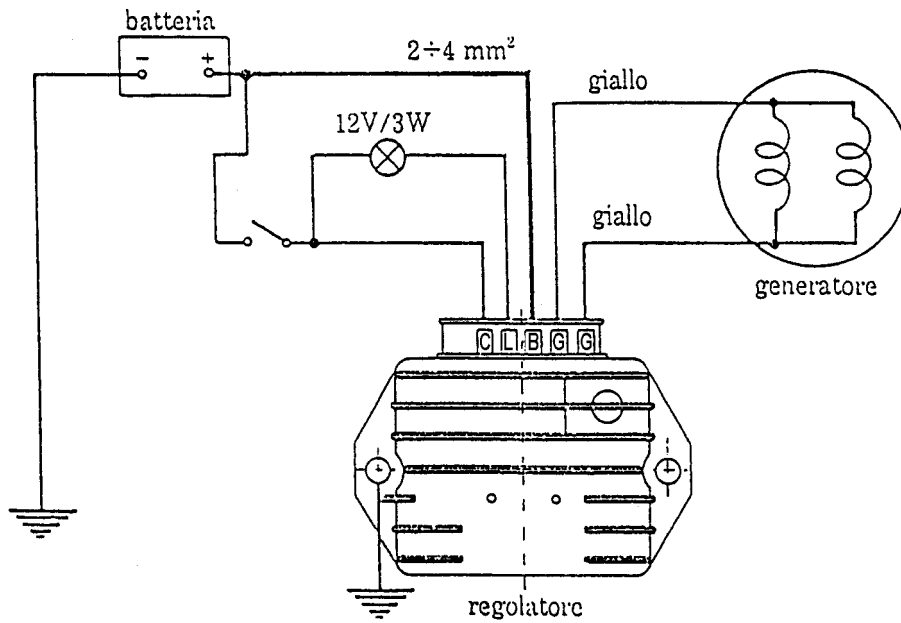
Schema d'inserzione dei regolatori "a ponte" dotati di circuito spia (L) per lampadina segnalatrice di carica
